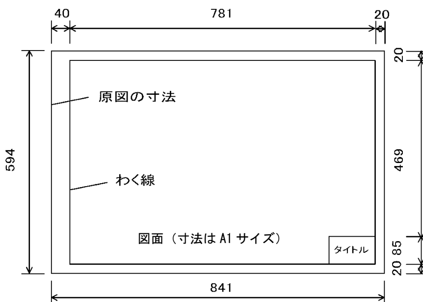
図-1 図面寸法 (単位mm)
